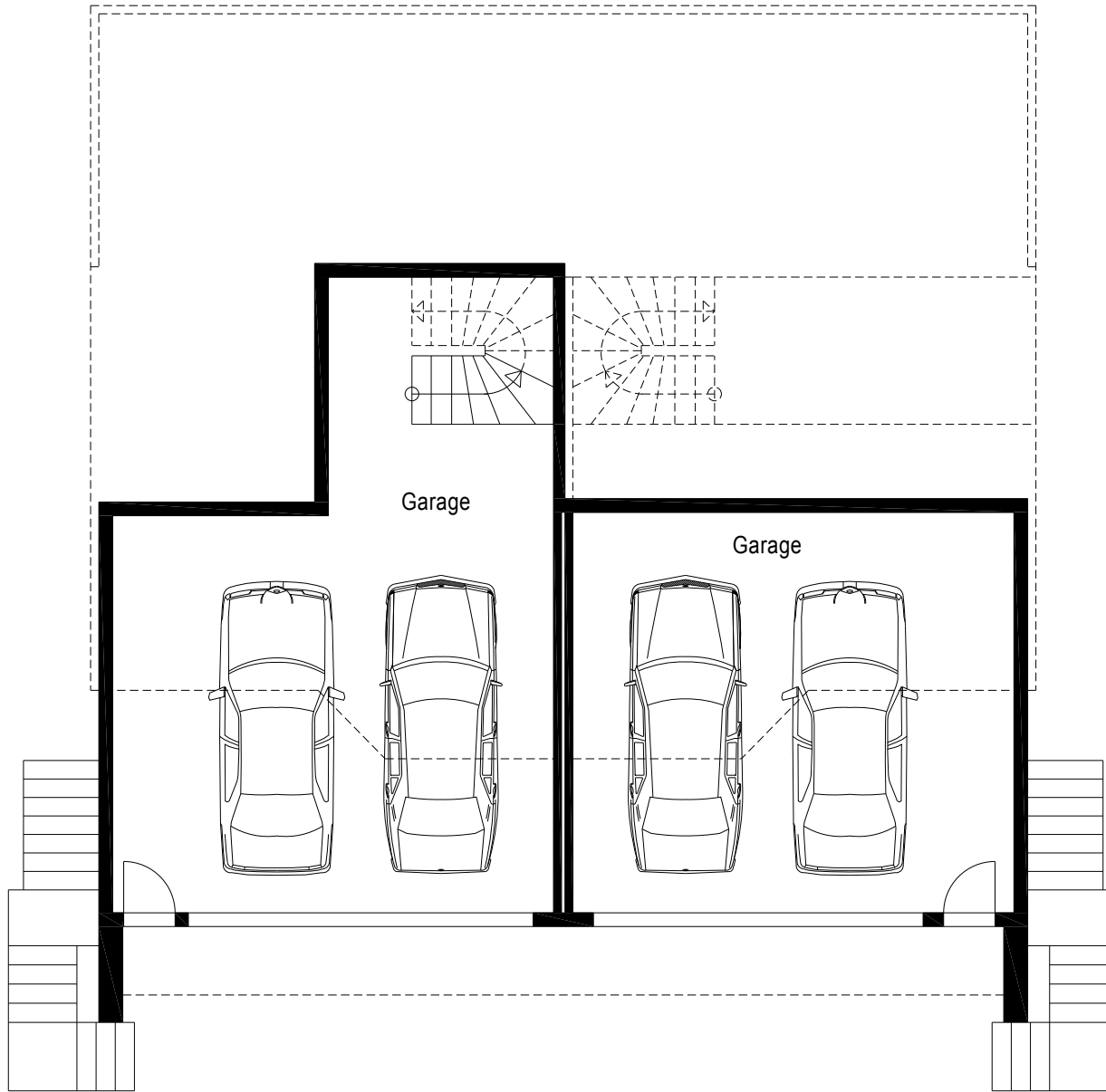
Garagengeschoss
